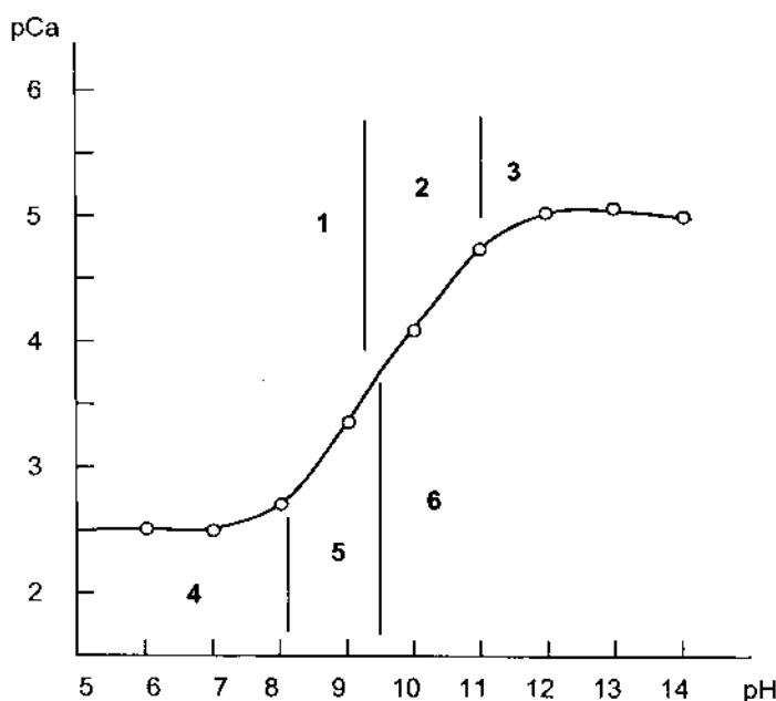
Hình 10.9. Giải đồ phân bố đối với dung dịch murexid khí có ion calci
