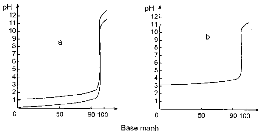
Hình 7.17. Trung hoà: a) một acid mạnh bằng 1 base mạnh. b) một acid yếu bằng 1 base mạnh.
